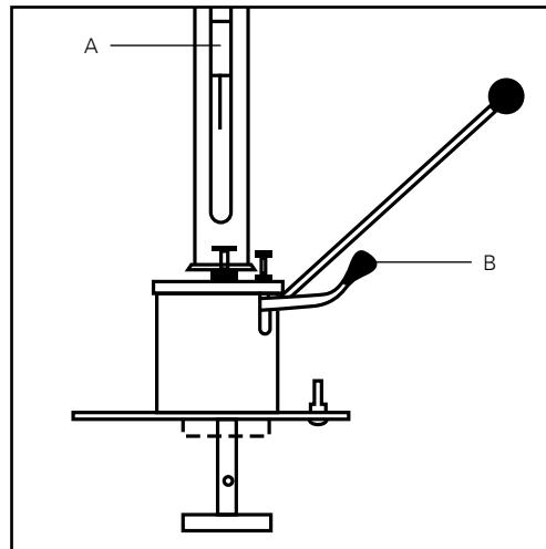
Fig. 4 Perskop onder tegen de machinekop aanzetten
