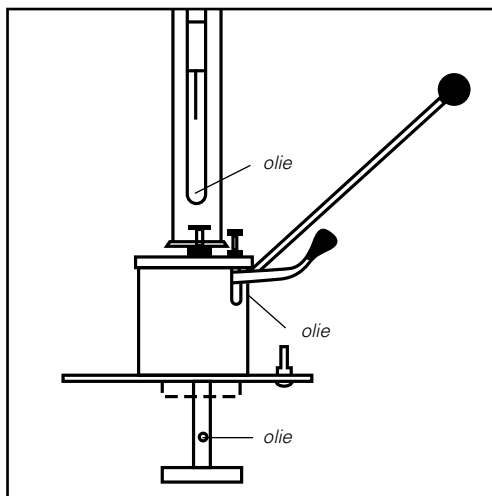
Fig. 10 Regelmatig olie aanbrengen voor een langere levensduur van uw Ras®-patatmachine
